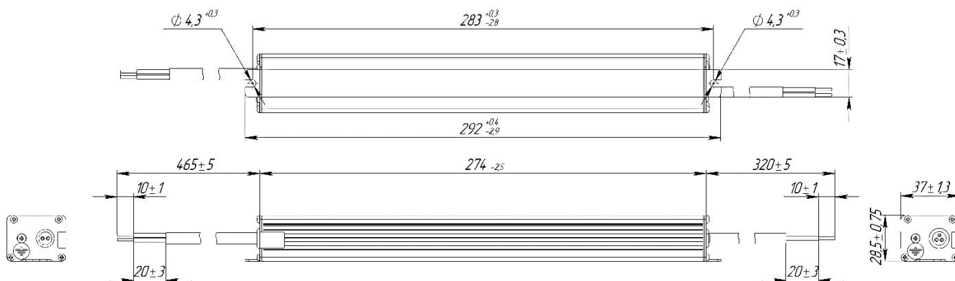
Рисунок 1 – Габаритные и установочные размеры
